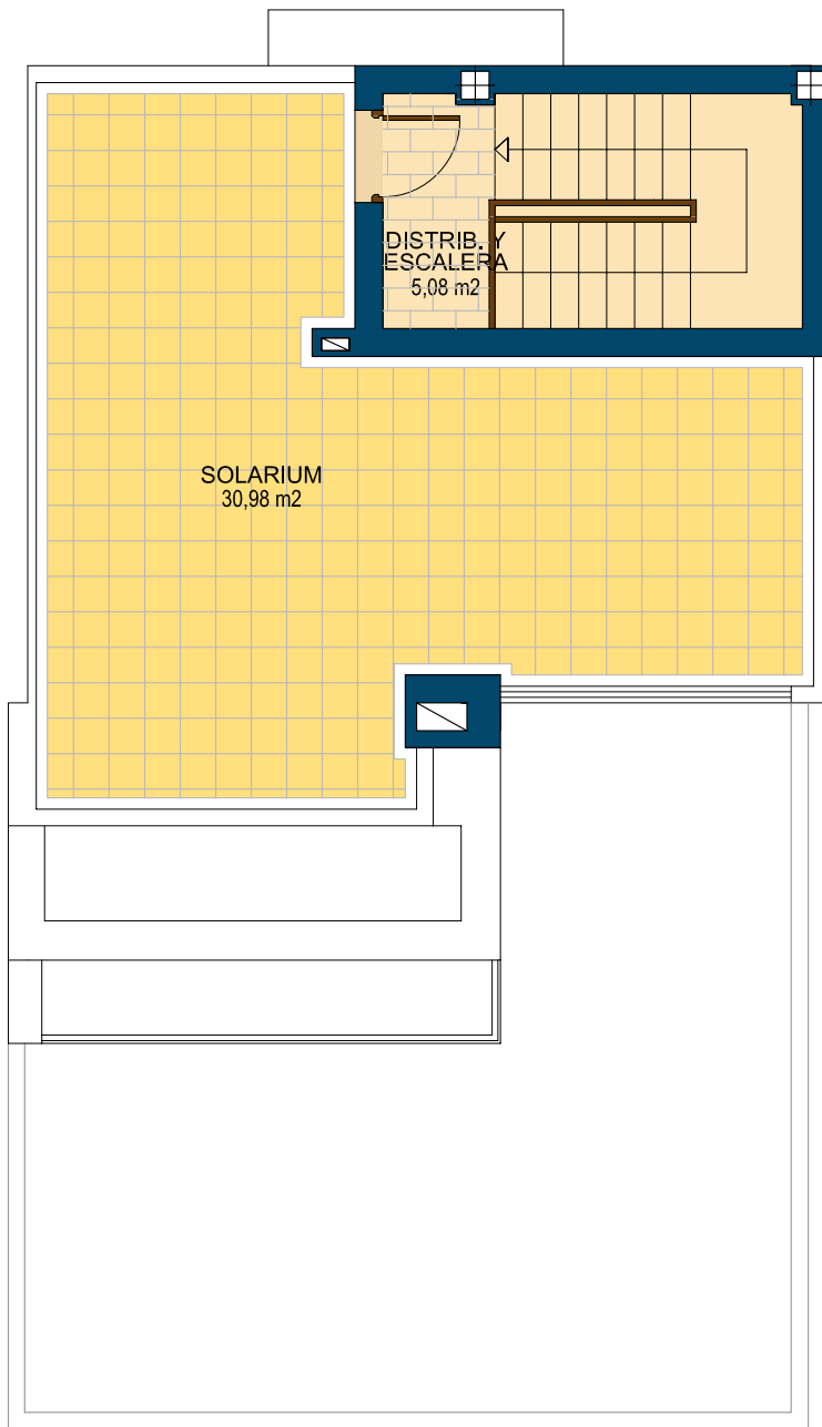
PLANTA SOLARIUM
